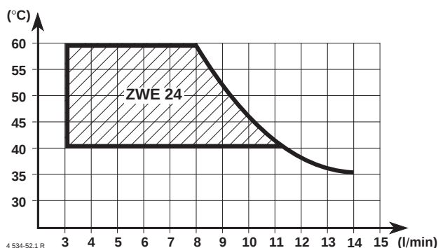
Fig. 54 Diagramma portata acqua calda sanitaria
