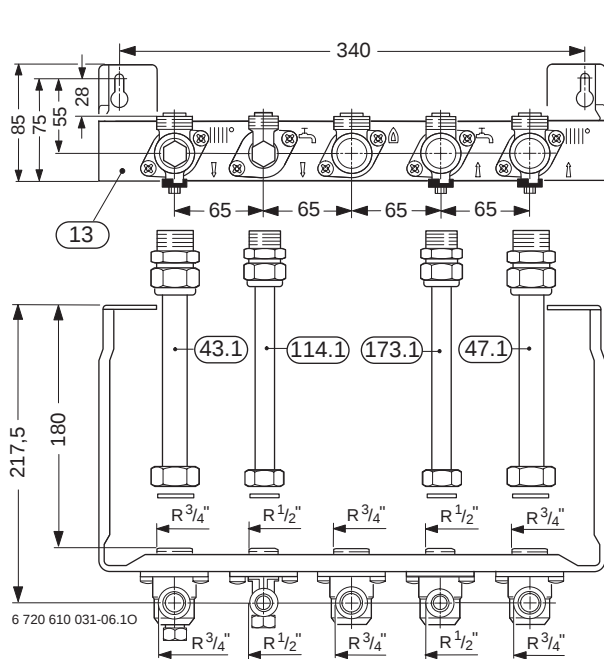
Fig. 7 Piastra di allacciamento e di montaggio - come viene fornita
